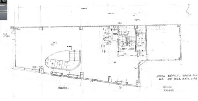
2階 平面図
